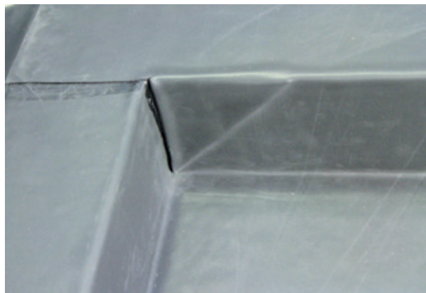
Aspect de finition d'un angle intérieur avant la finition de la partie supérieure du relevé.
