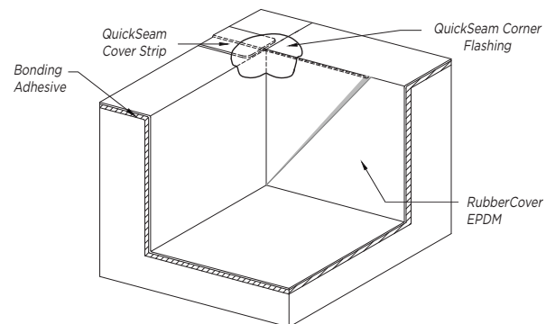
Finition de la partie supérieure d'un angle intérieur avec une pièce QuickSeam Corner Flashing et une bande QuickSeam Cover Strip.
